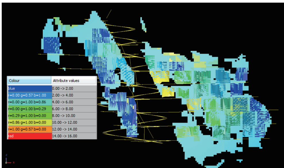
圖2－Nevoria East地下金礦地下開發簡圖
